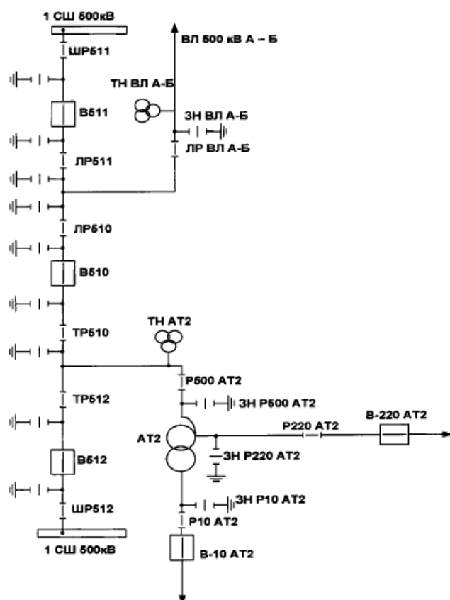
Рисунок 3. Схема ПС 500 кВ, выполненная по полуторной схеме
