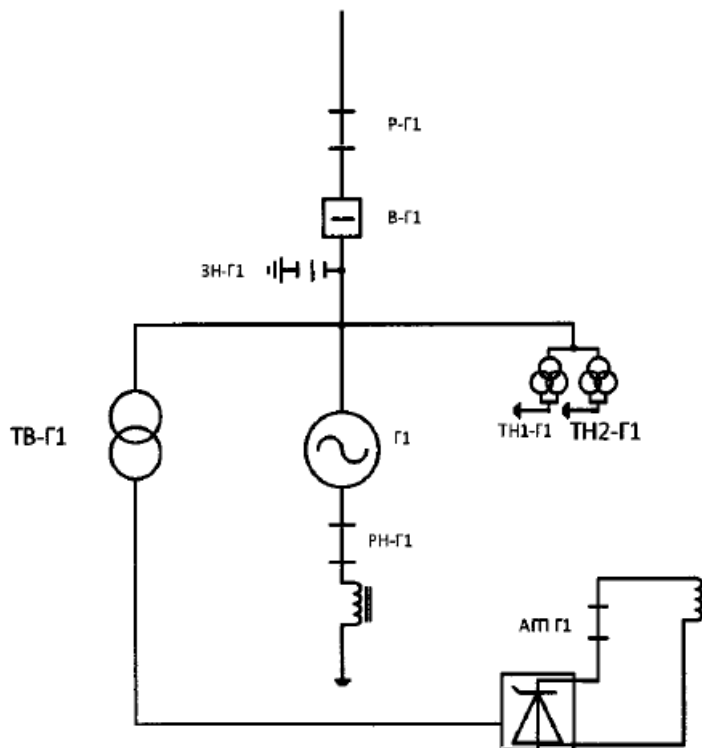
Рисунок 2. Нормальная схема генератора Г1
