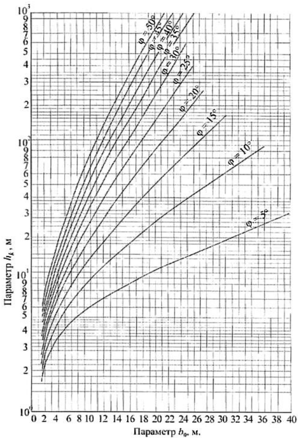
Рисунок В.6 - Графики для определения параметра b_0
