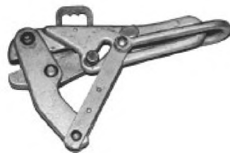
Натяжной клиновой зажим для заземляющего проводника
