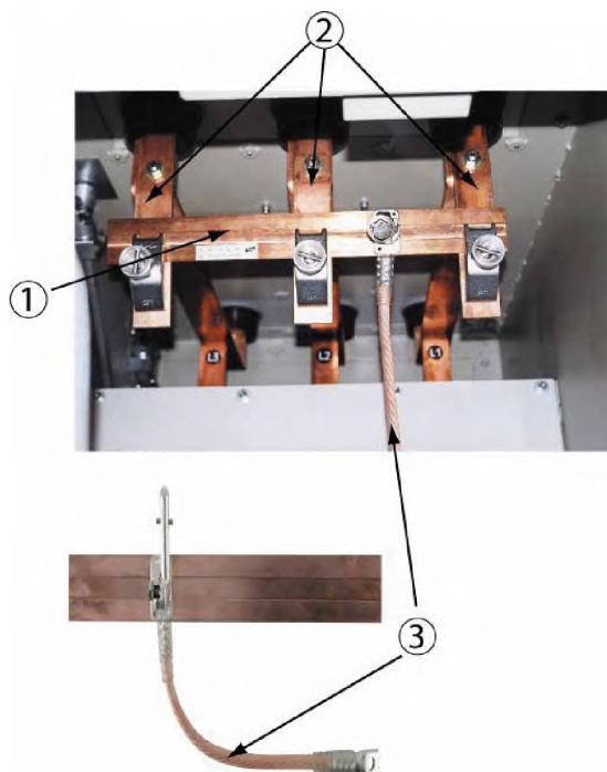
1 — короткозамыкающая шина; 2 — проводники; 3 — кабель заземления
