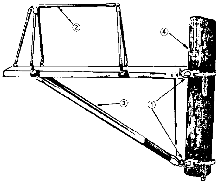
1 — цепная стяжка; 2 — вспомогательный поручень; 3 — кронштейн; 4 — опора
