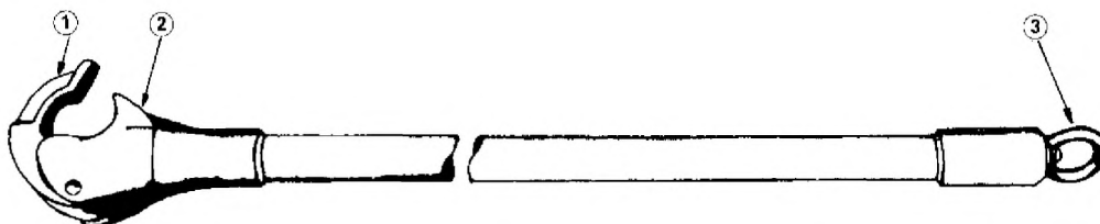
1 — подвижная челюсть; 2 — неподвижная челюсть; 3 — поворотное кольцо
