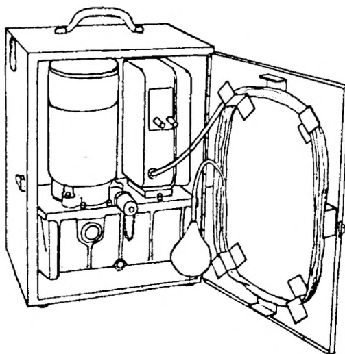
Гидравлический агрегат с электродвигателем
