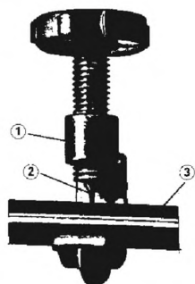
1 — винт; 2 — металлический наконечник винта; 3 — изолированный проводник
