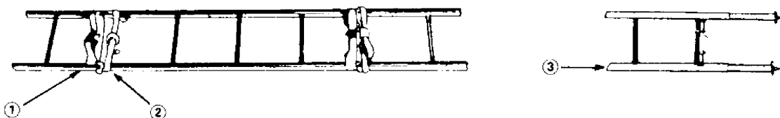
1 — стойка (рельс); 2 — привязной ремень; 3 — нижняя секция (с регулируемыми опорами)
