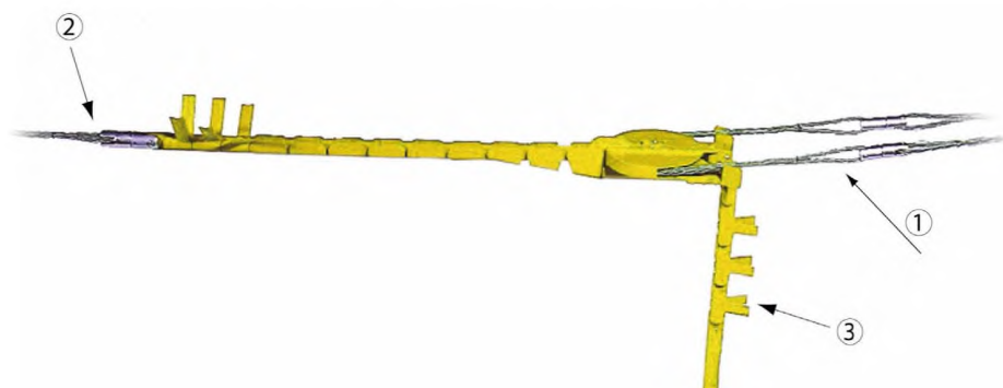
1 — провод; 2 — протягиваемый трос; 3 — хвостовик
