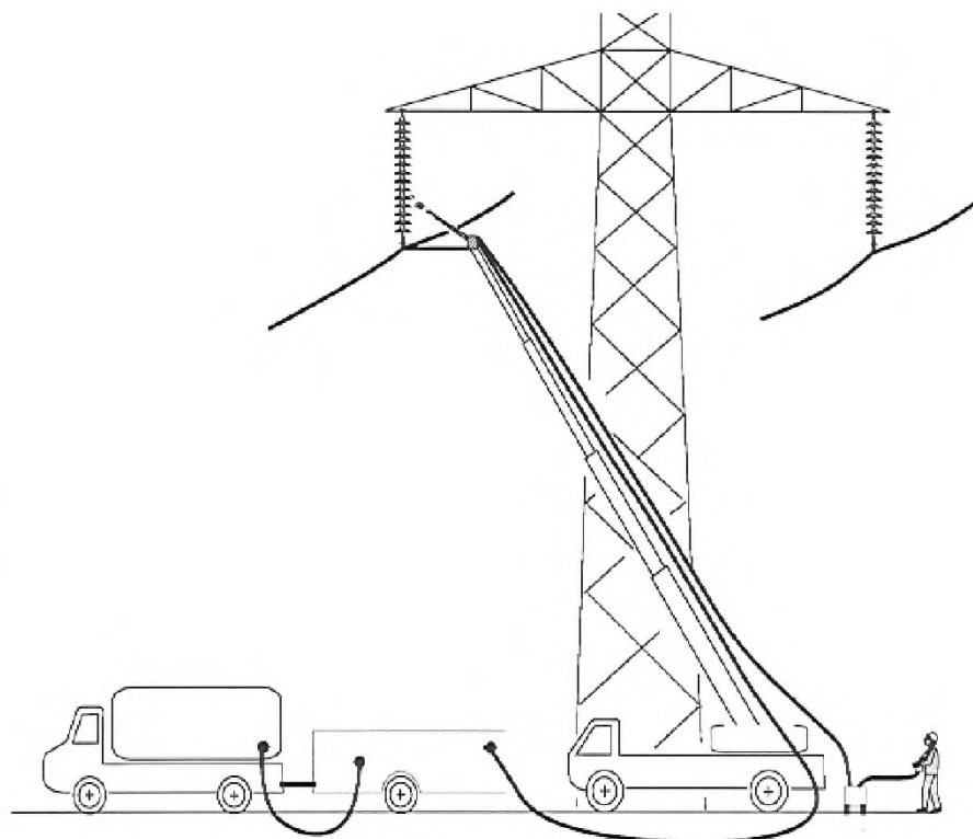
Оборудование для влажной чистки водой под давлением
