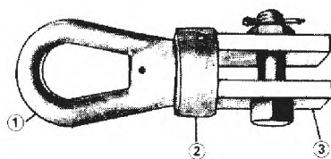
1 — ушко; 2 — вертлюг; 3 — вилка
