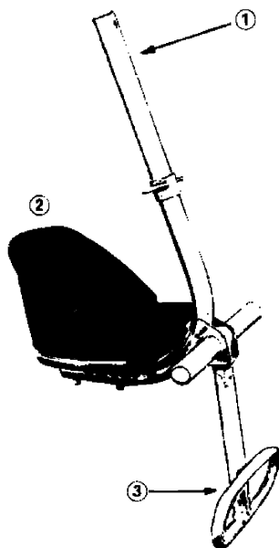
1 — штанга для крепления; 2 — сиденья; 3 — упор для ног
