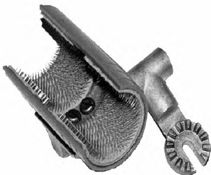
Полутрубчатая щетка
