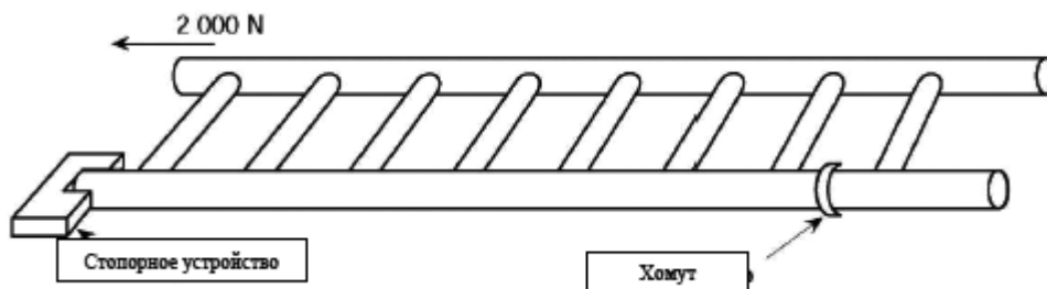
Рис.8. Испытания перекладин/тетив в сборе Электрические испытания лестницы по истечении срока службы
