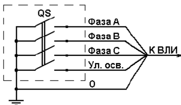
Рис.13. Схема стационарного устройства заземления
