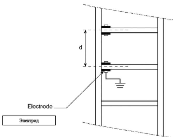
Рис.9. Схема электрических испытаний
