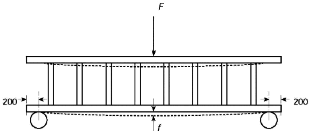
Рис.5. Испытания на боковой прогиб
