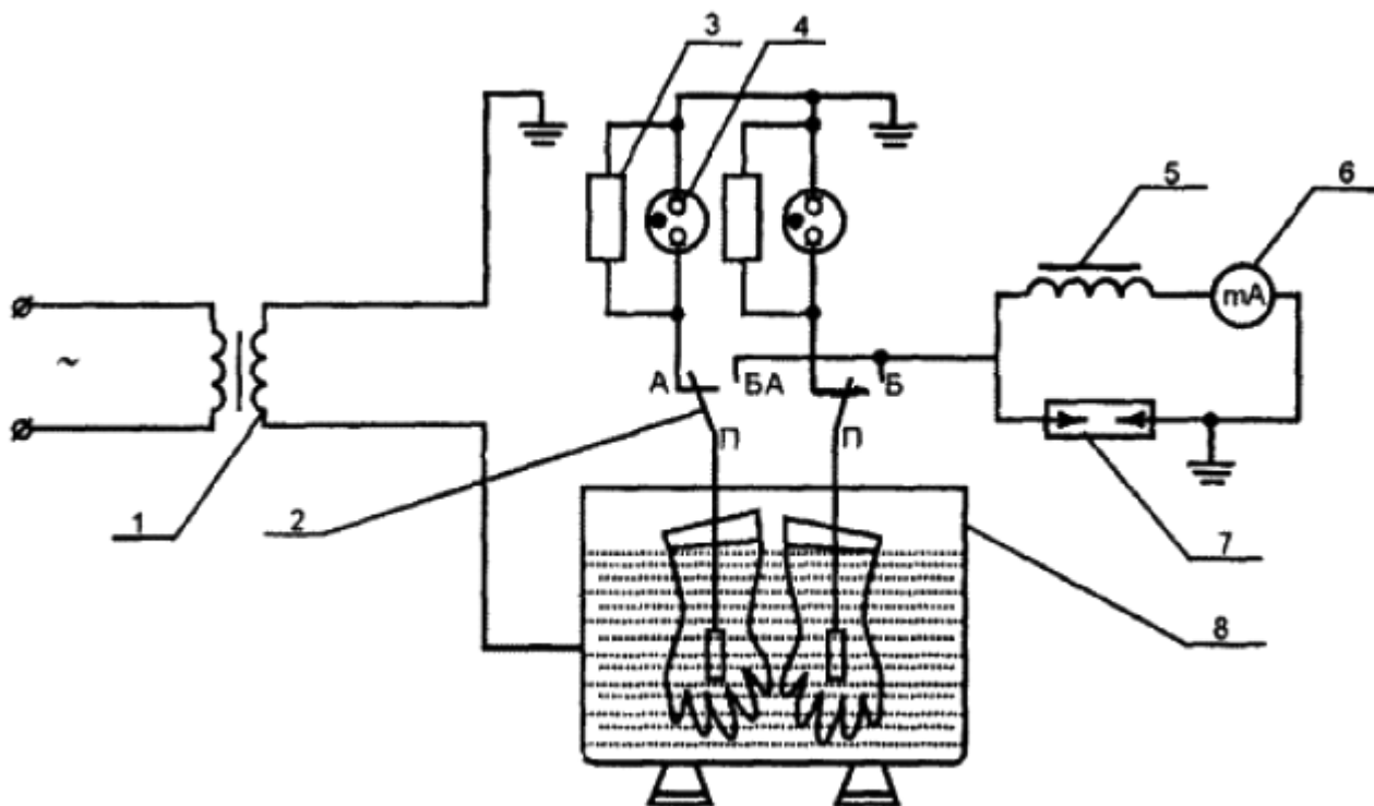
Рис.11. Принципиальная схема испытания диэлектрических перчаток:
