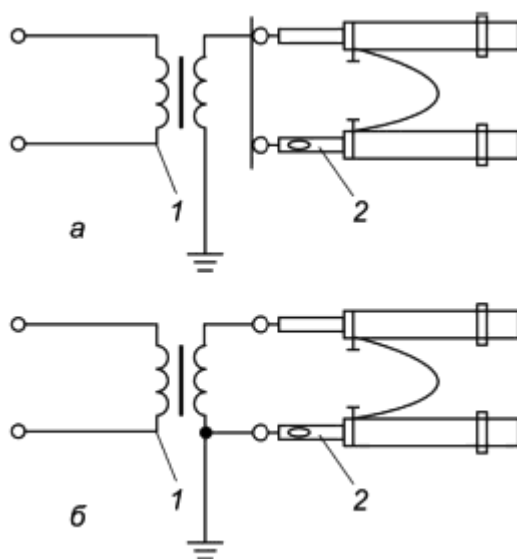
Рис.2. Принципиальные схемы испытания указателя напряжения для проверки совпадения фаз по схеме согласного (а) и встречного (б) включения
