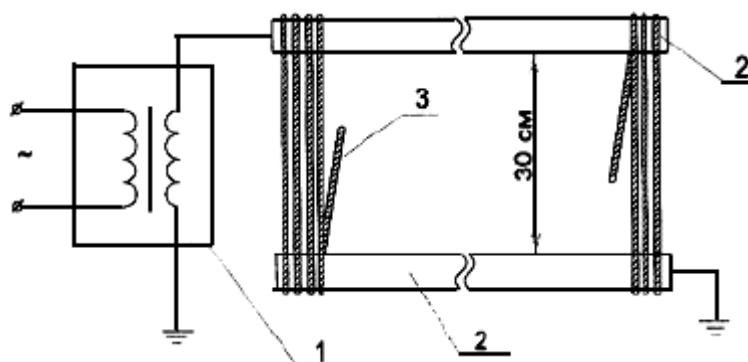
Рис.3. Схема электрических испытаний изолирующего каната:
